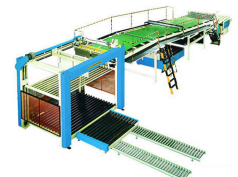
DOWN STACKER Empilhador automático
